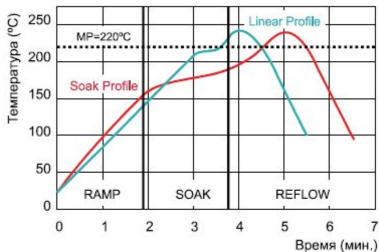
Рис. Рекомендуемый профиль для сплава SAC0307
