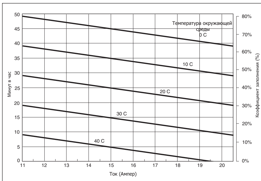
Рисунок 5. Допустимая длительность тока &gt;11 А
