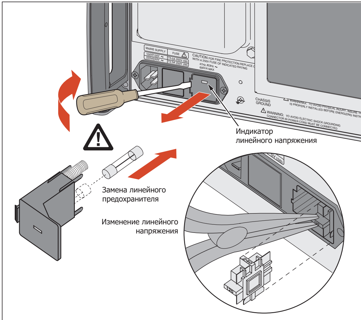
Рисунок 3. Доступ к предохранителю и выбор сетевого напряжения
