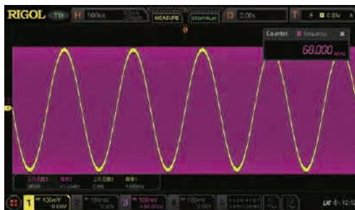
Измерение частоты встроенным частотомером
