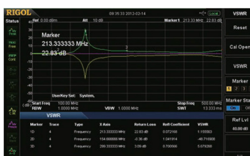
Программное обеспечение для ПК
