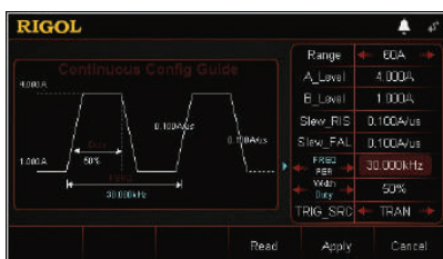
30 кГц динамический режим
