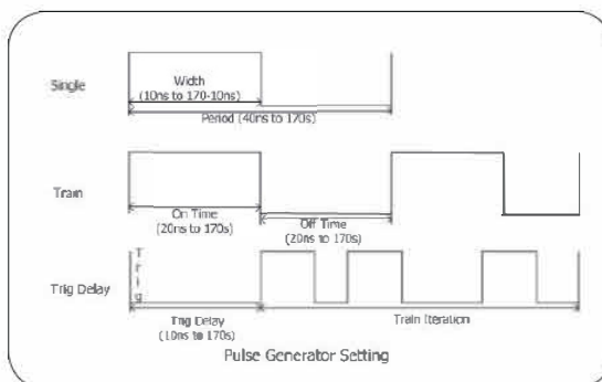
Импульс, (опция)
