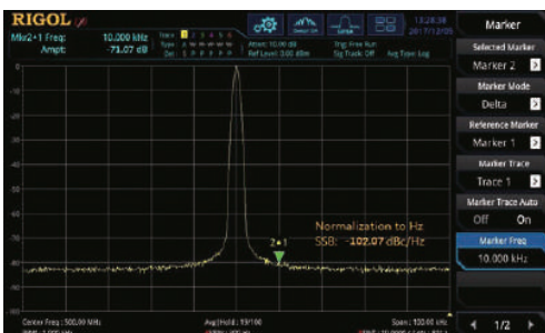
Уровень фазовых шумов -102 дБн/Гц
