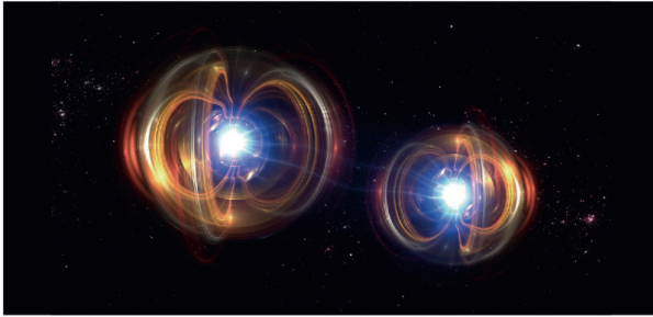
Сверхпроводящие квантовые вычисления
