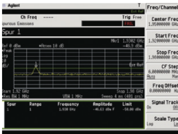
Испытания аппаратуры по техническим требованиям 3GPP W-CDMA TS21.141 на уровень побочных излучений
