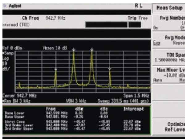
Интермодуляционные искажения двухчастотного сигнала
