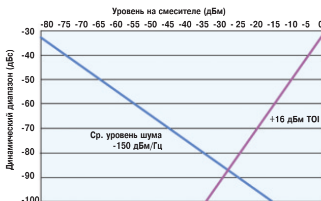
Выдающиеся характеристики по интермодуляционным искажениям третьего порядка обеспечивают максимальный динамический диапазон
