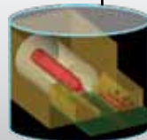
Импорт CAD-файла
