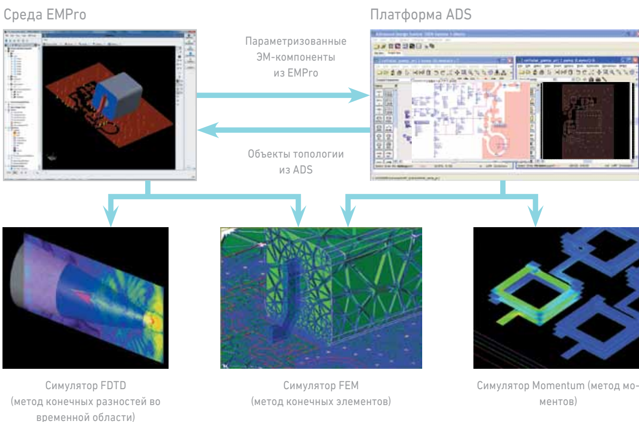
Рис. 1. Компания Keysight предоставляет несколько технологий ЭМ моделирования, интегрированных в маршрут проектирования в САПР ADS.
