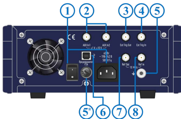
Рисунок 4.6 Задняя панель
