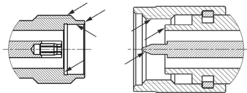
Рисунок 3.2 Соединители тип 3,5 мм и IX (розетка и вилка)
