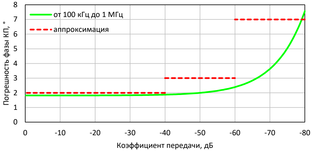
Погрешность измерений фазы коэффициента передачи согласованных устройств анализаторов С1214, С1220, С1420, С2220 С2420, С4220, С4420
