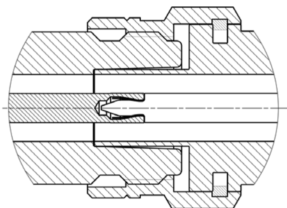
Рисунок 3.5 Соединители тип N и III (розетка слева, вилка справа)
