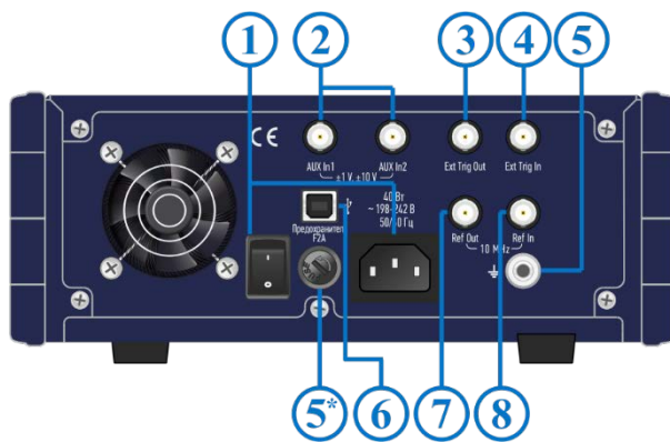
Рисунок 4.4 Задняя панель
