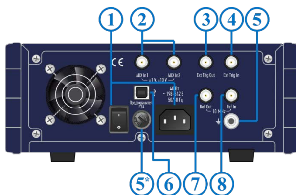
Рисунок 4.2 Задняя панель
