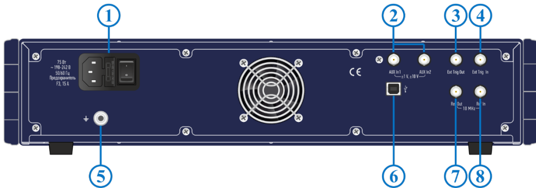
Рисунок 4.12 Задняя панель
