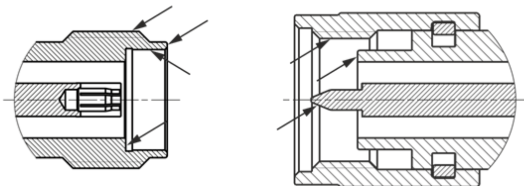
Рисунок 5 – Соединители тип 3,5 мм или IX (розетка и вилка)
