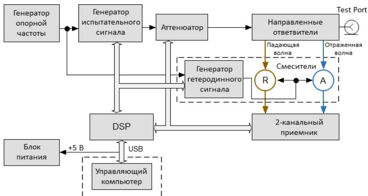
Рисунок 2 – Функциональная схема рефлектометра
