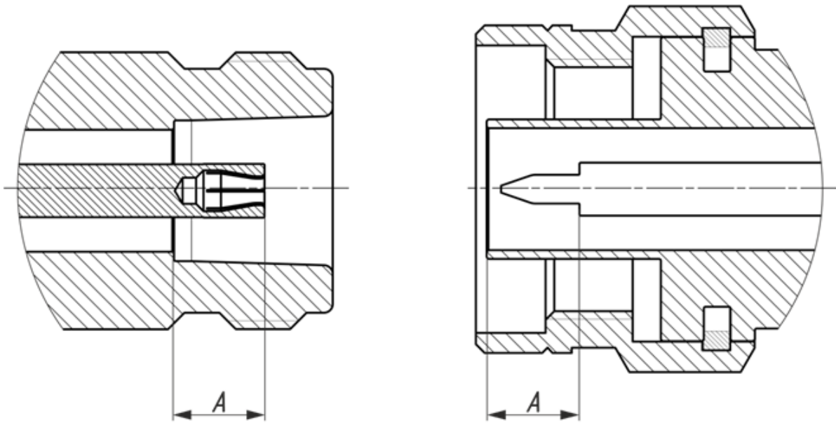
Рисунок 6 – Соединители тип N (розетка и вилка)
