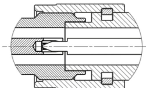
Рисунок 9 – Соединители тип 3,5 мм (розетка слева, вилка справа)
