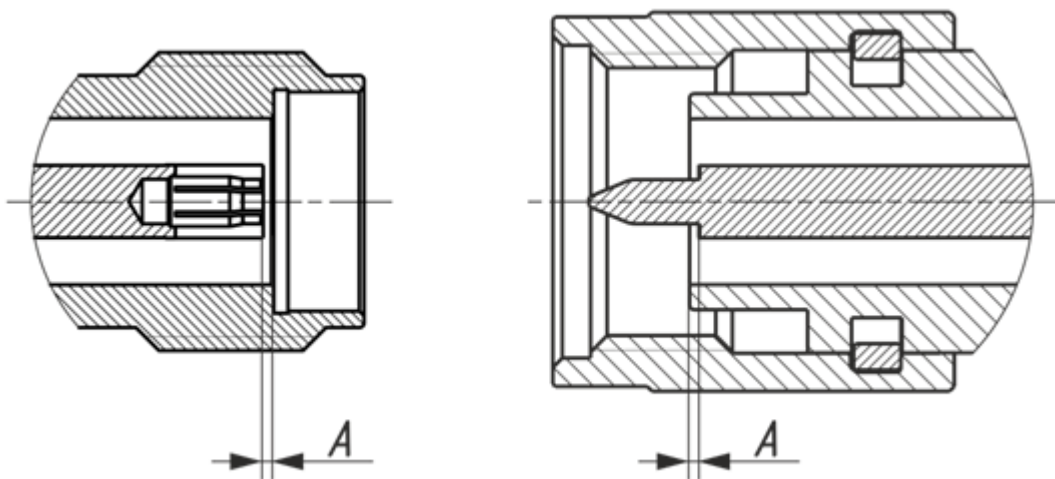
Рисунок 7 – Соединители тип 3,5 мм (розетка и вилка)
