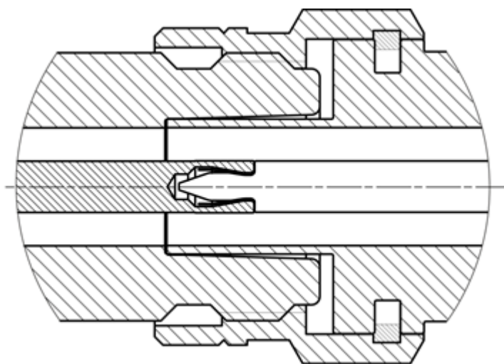
Рисунок 8 – Соединители тип N (розетка слева, вилка справа)
